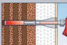
6. Заполнить отверстие составом FIS V.
