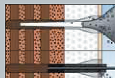
4. Продуть отверстие.
