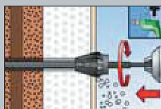
3. Вкрутить Thermax
