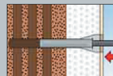
5. Вставить перфорированную гильзу.
