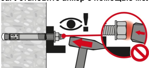
4. Проверьте корректность установки анкера
