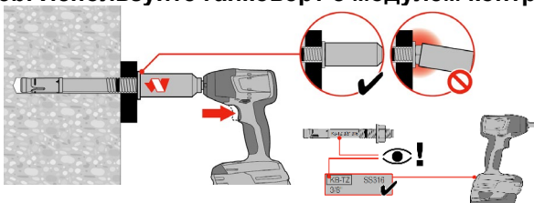
5б. Используйте гайковерт с модулем контроля затяжки (M8-M12)
