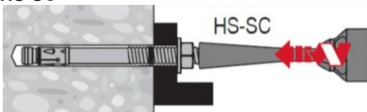
2б. Используйте установочное устройство HS-SC
