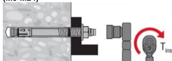
5.а Приложите требуемый момент затяжки (M8-M24)
