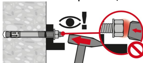
3. Проверьте корректность установки анкера
