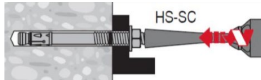
3б. Используйте установочное устройство HS-SC
