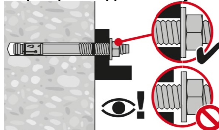
3. Проверьте корректность установки анкера
