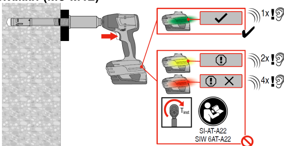
5б. Используйте гайковерт с модулем контроля затяжки (M8-M12)
